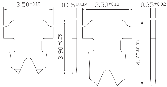
2 PRONGS FOR STRANDED WIRE 多芯線用二叉型片
