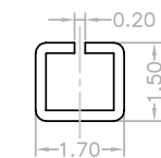
SEC:D-D
