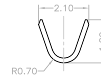
SEC:B-B
