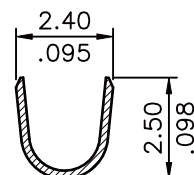
SEC:A-A
