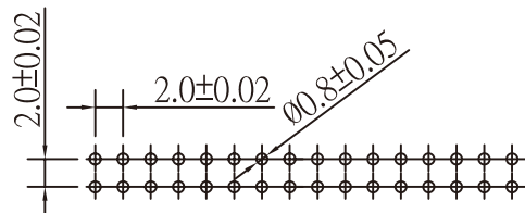
P.C.Board Layout
