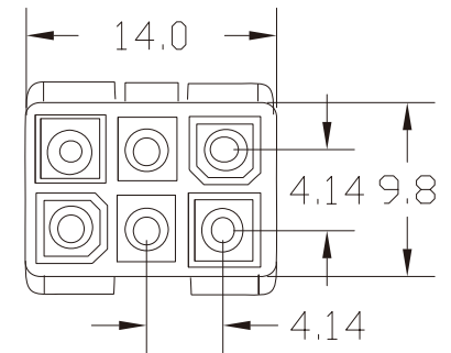
ML-P-2X03
