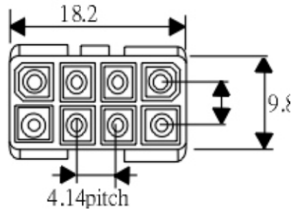
ML-P-2X04
