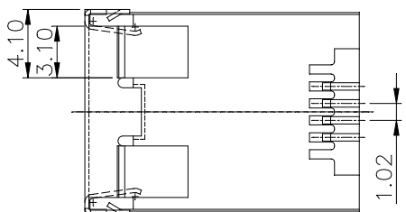
成品上PCB板情形
