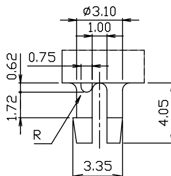
DETAIL Y
