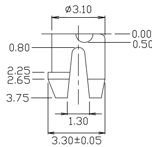
DETAIL Y
