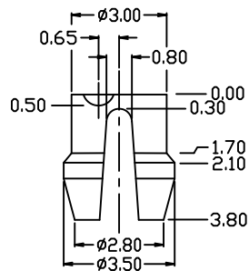
DETAIL Y
