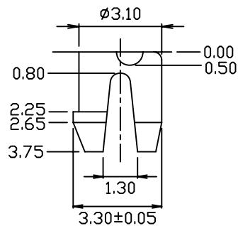
DETAIL Y
