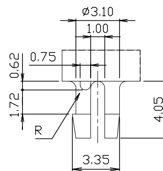
DETAIL Y
