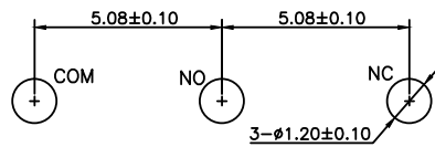
P.C.B LAYOUT
