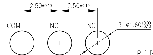
P.C.B LAYOUT
