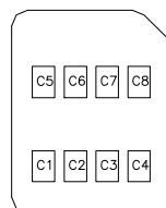
【 SIM CARD PAD LAYOUT 】
