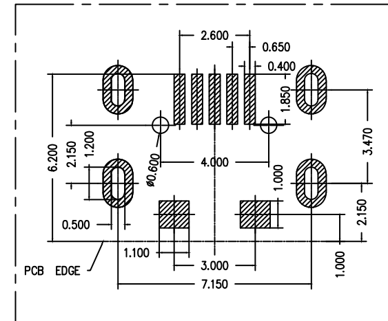
PCB参考图
