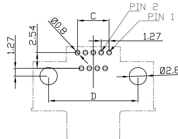
P.C.B. LAYOUT
