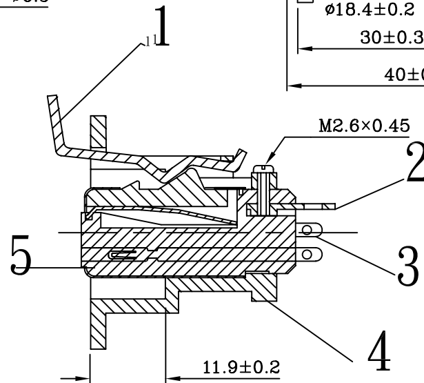
A-A SECTION
