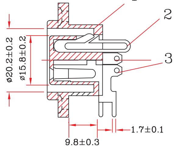
A-A SECTION
