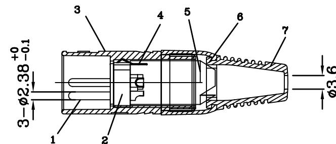
A-A SECTION
