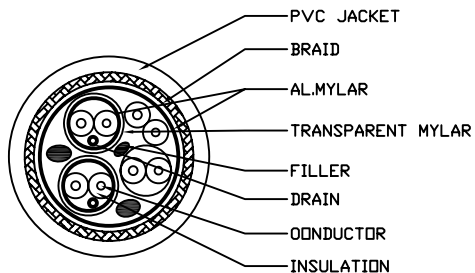
SEC A-A
