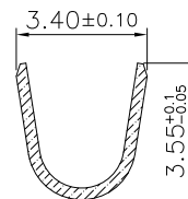
SECTION A-A SCALE 2:1
