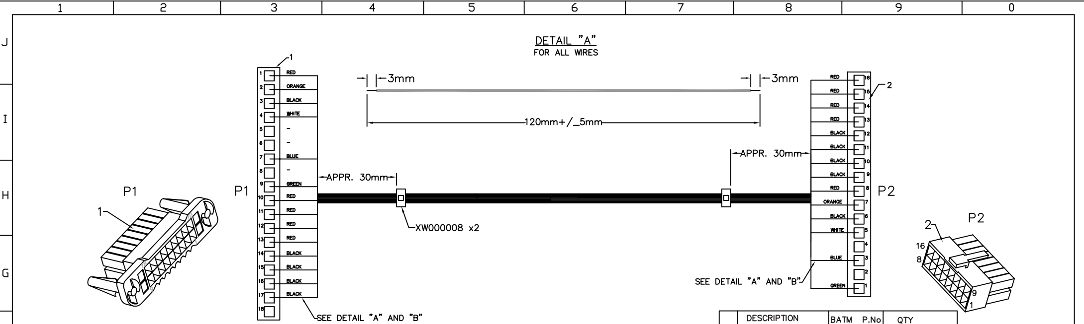
WIRING TABLE
