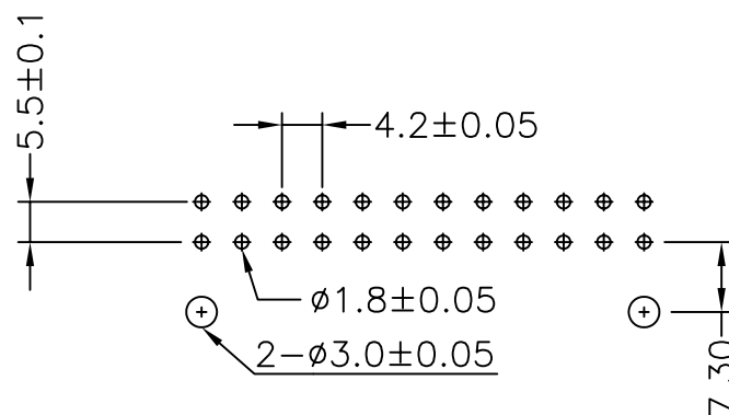
P.C.B. LAYOUT
