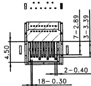
剖面圖 A-A
