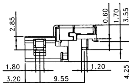
剖面圖 A-A
