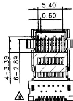
剖面圖 B-B
