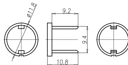
POM RING
