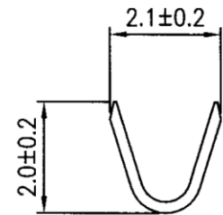
A-A SECTION
