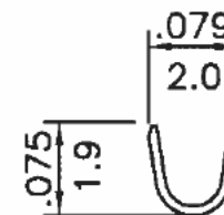
A-A SECTION
