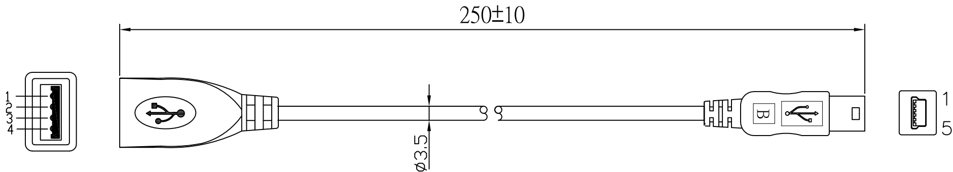
P2 MINI USB 5P B TYPE
