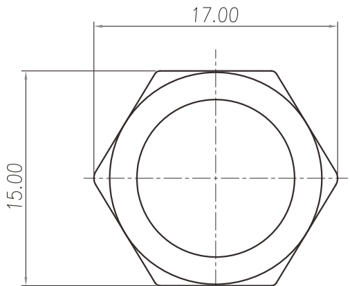
NUT
