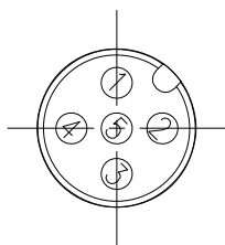
端子排位 正视图
