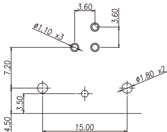
P.C.B LAYOUT 8P
