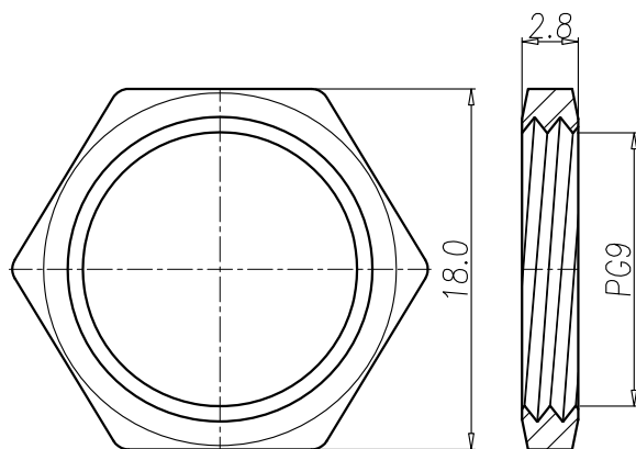
NUT
