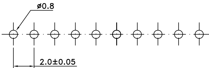
P.C.B. LAYOUT
