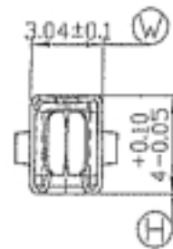
SEC.B-B
