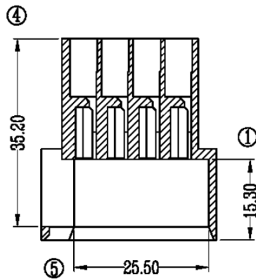
SEC:A-A
