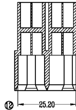
SEC:B-B
