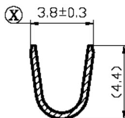
SEC. A-A
