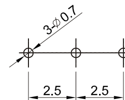
P.C.B LAND PATTERN
