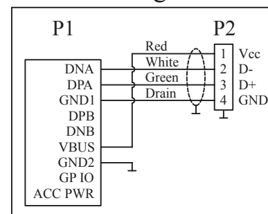
Wiring Table
