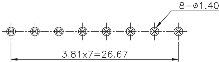
P.C.B LAYOUT
