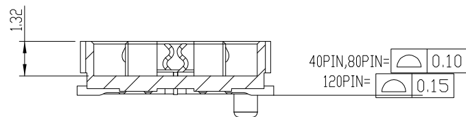
剖面圖 A-A
