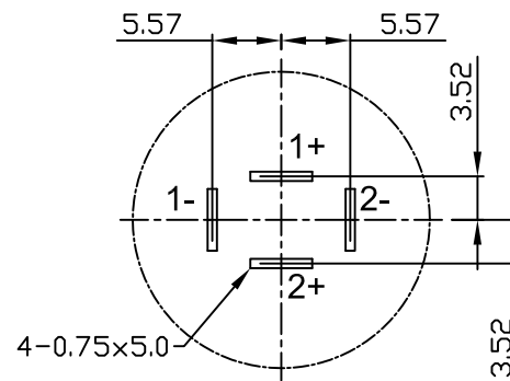
△ P.C.B LAYOUT(±0.1)
