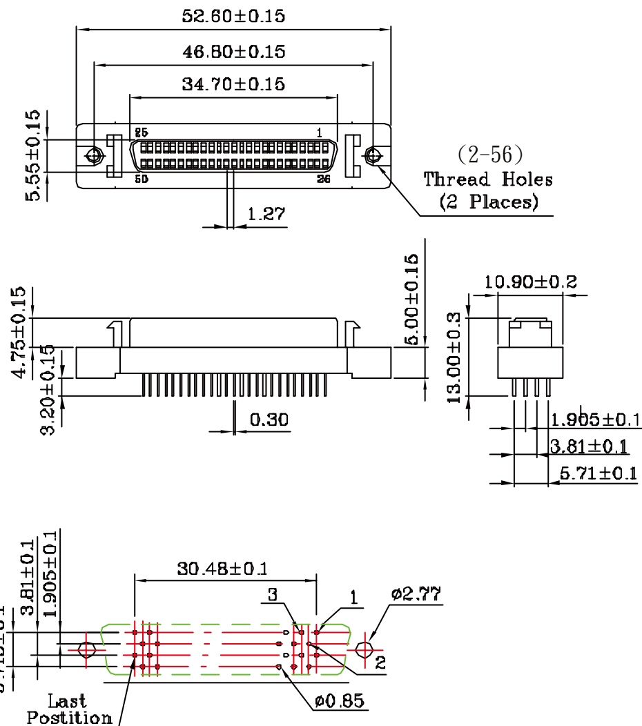
P.C.Board Hole Pattern
