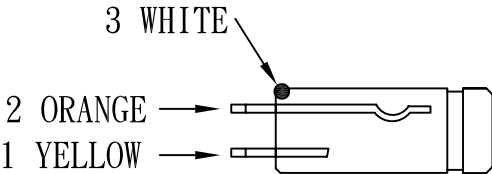
焊接示意圖
