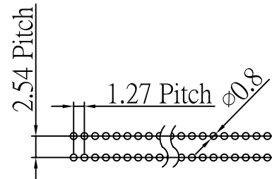
P.C.Board Layout
