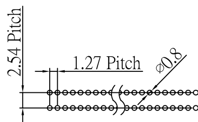
P.C.Board Layout
