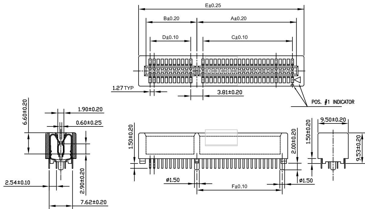
SECTION A-A
