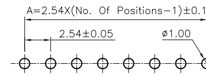
P.C.B. Layout
