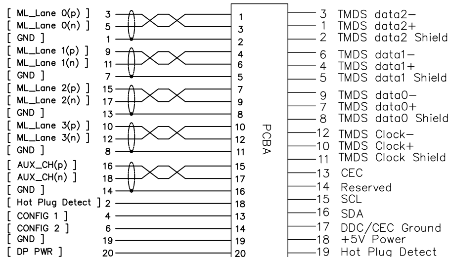
MINI DP PLUG (SOURCE)
