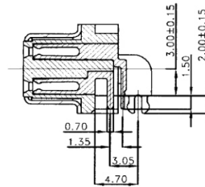
A-A SECTION
