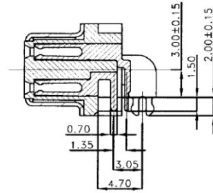
A-A SECTION
